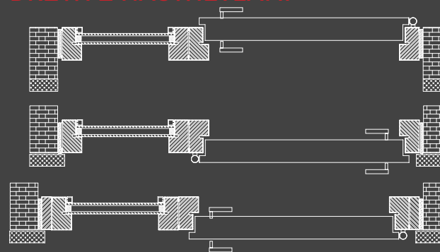
drzwi otwierane do wewnątrz z ościeżnicą symetryczną
