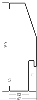
OŚCIEŻNICA PD56/150
